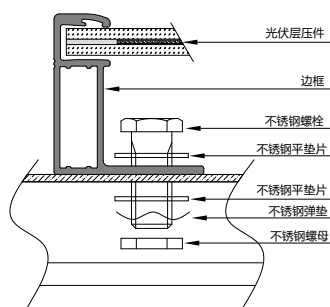
图10：螺栓结构图
