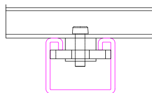
图12：预固定压块
