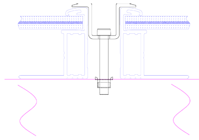
图13：拧紧压块
