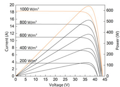
I-V / P-V CURVES
