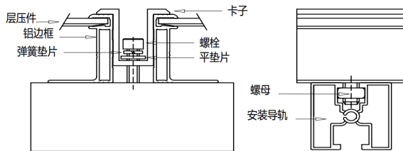
图13：压块安装方式明细
