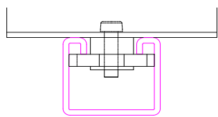
图18：预固定压块
