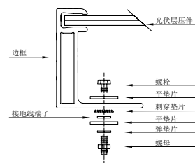
图10: 螺丝配合接地
