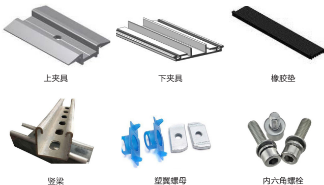
图12: 安装配件
