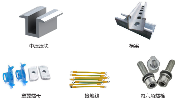
图17：安装配件
