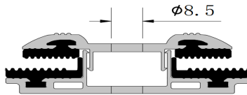
图11: 中压夹具
