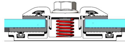
图13: 预固定夹具
