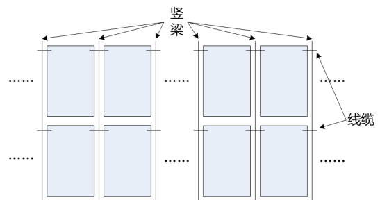
图15: 无框双玻组件方阵
