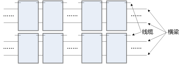
图14: 双玻组件方阵
