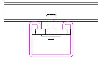
图12: 预固定压块
