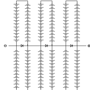
图7：电池片和旁路二极管的电路系统
