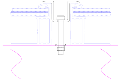
图13: 拧紧压块
