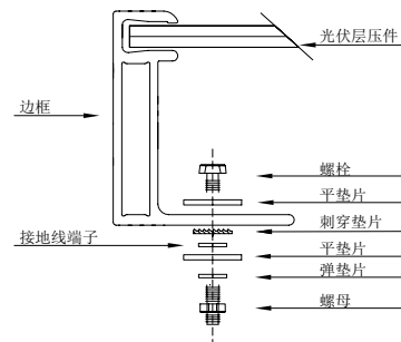
图10: 螺丝配合接地
