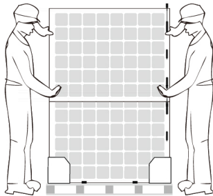
图3：无框双玻组件取出示意图
