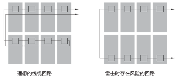
图5：线路设计
