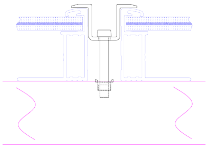
图19: 拧紧压块
