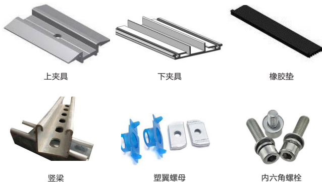
图12: 安装配件
