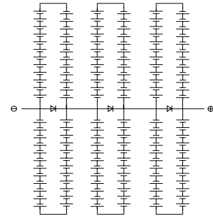
图8: 电池片和旁路二极管的电路系统
