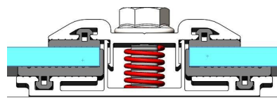
图13: 预固定夹具
