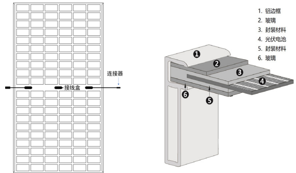
图1：双玻组件、横截面示意图
