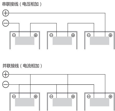
图6: 组件串并联电路图
