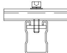
图14: 拧紧夹具
