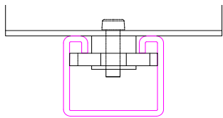
图18: 预固定压块
